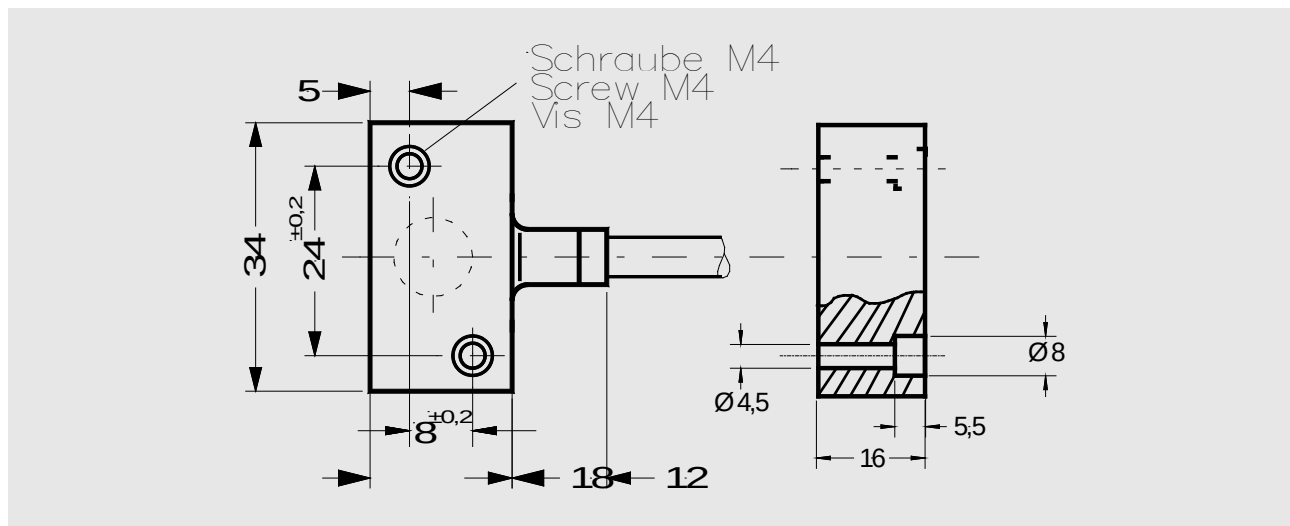
Abb. 1 Beschleunigungs-Sensor
