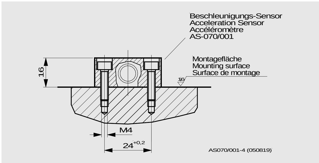
Abb. 4 Montage
